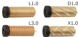
ストラクチャーローラー (替刃) L1.0 品番：4E50101 L3.0 品番：4E50104 L2.0 品番：4E50102 X1.0 品番：4E50143 D1.0 品番：4E50103 X2.0 品番：4E50144 各 ¥12,100 [ 税抜価格 11,000 円 ]
